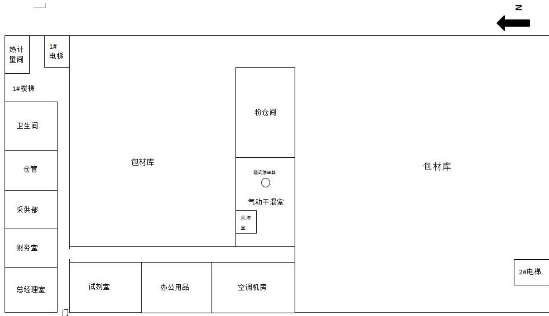
二层（车间设备设施布置图）
