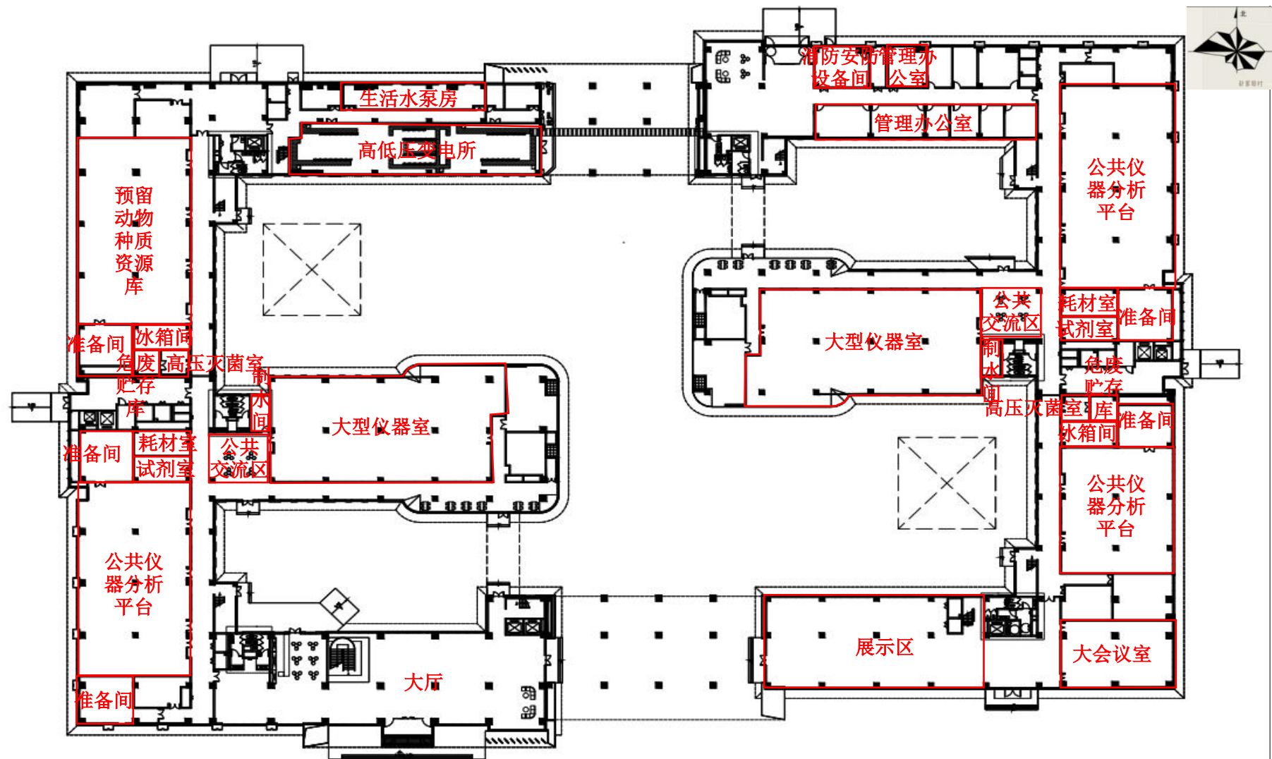
附图 5-1 一层平面布置图 (1:150)
