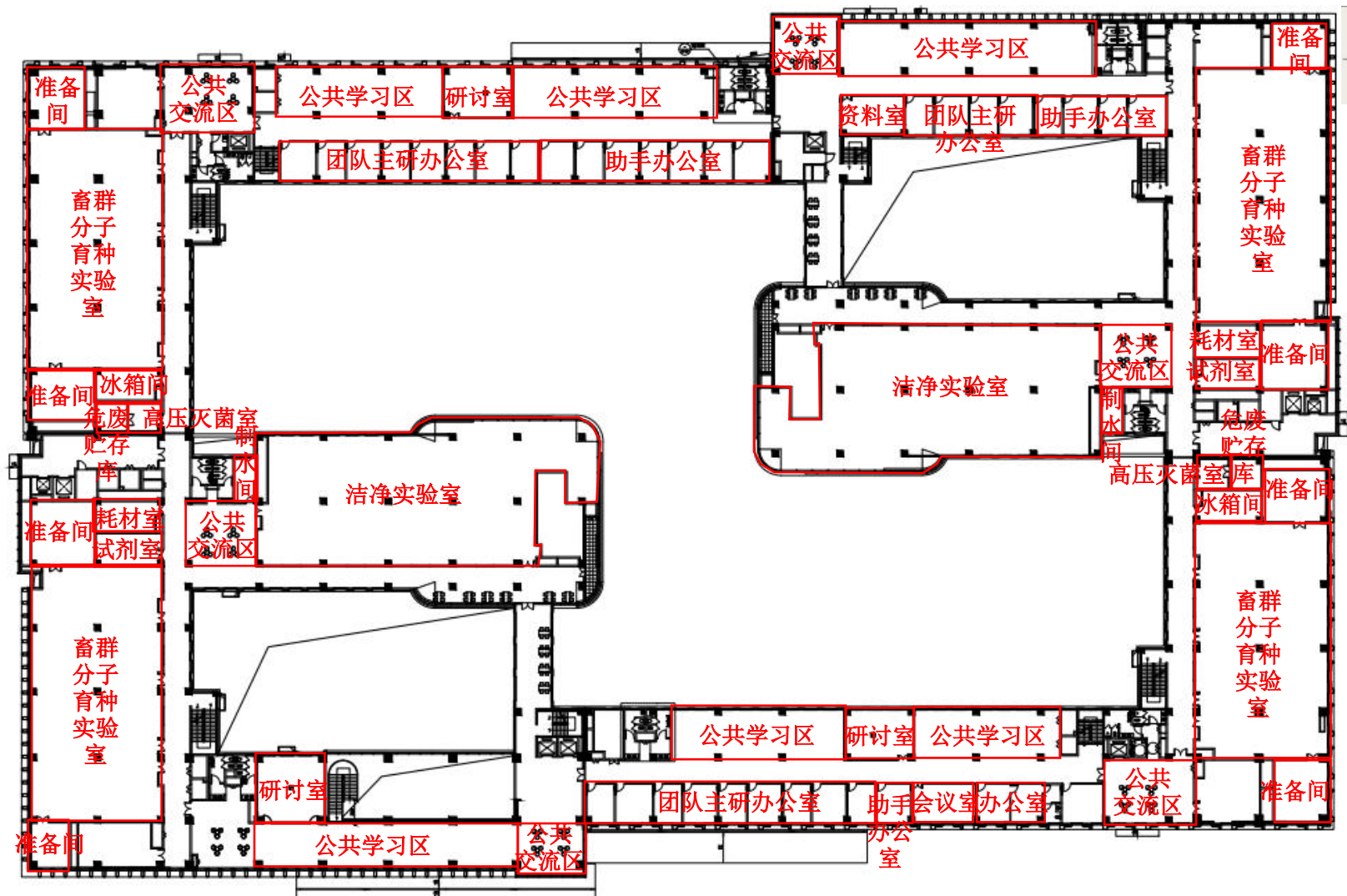
附图 5-2 二层平面布置图 (1: 150)
