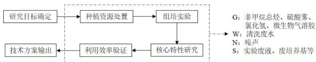
图 2-5 实验工艺流程及产污环节图
