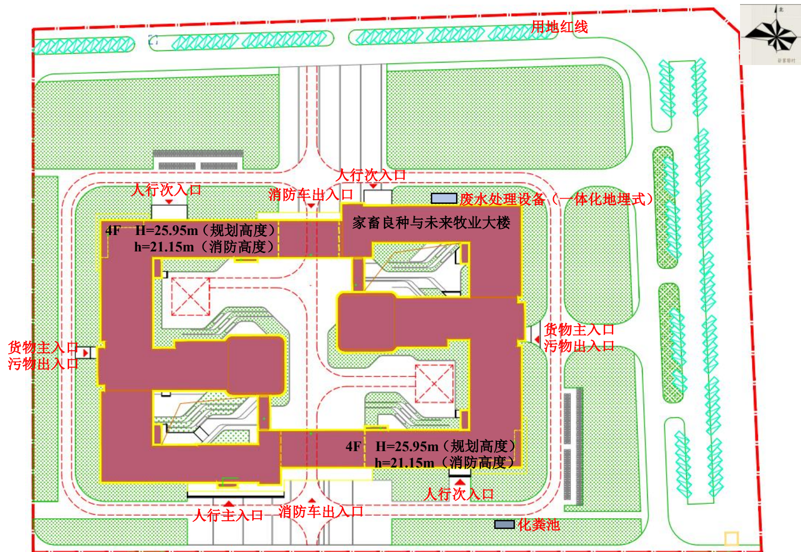
附图4 总平面布置图 (1:500)
