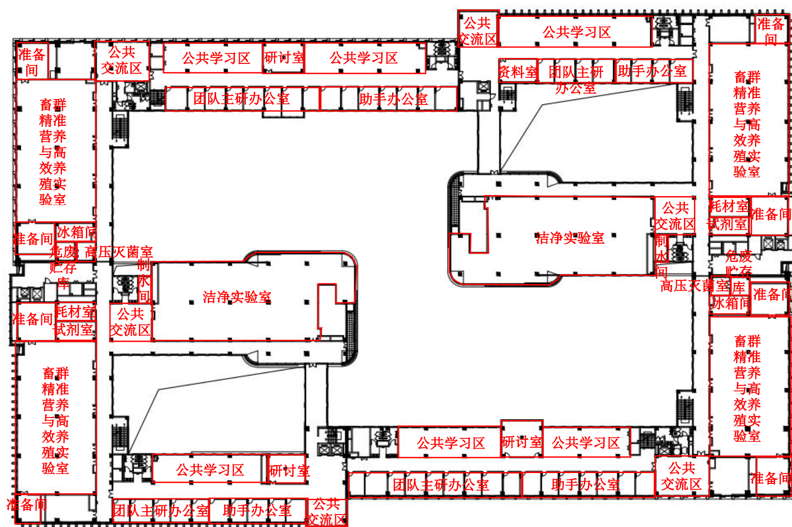
附图 5-3 三层平面布置图 (1:150)
