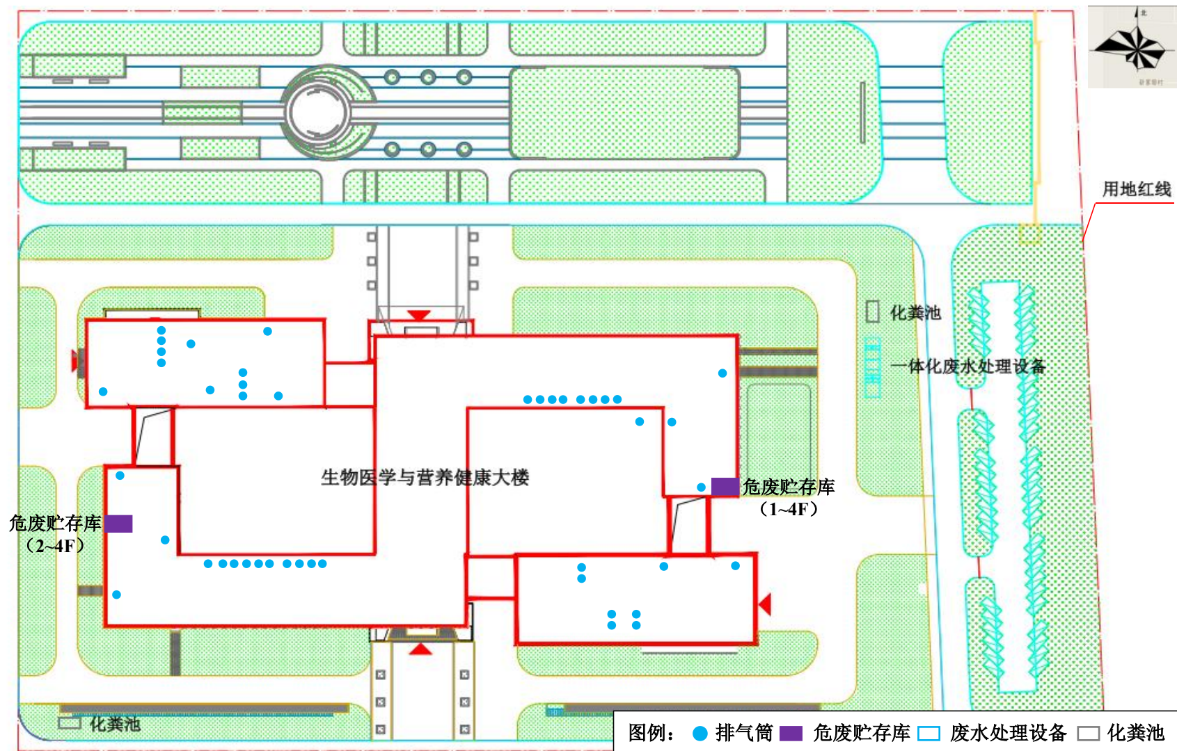
附图 6 环保设施位置图 (1:500)
