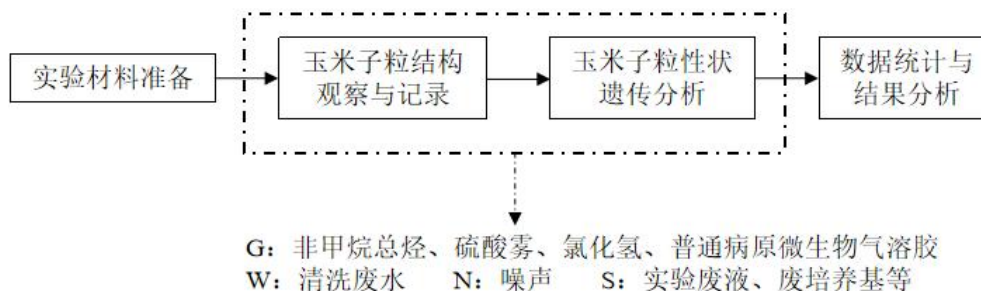
图 2-3 实验工艺流程及产污环节图
