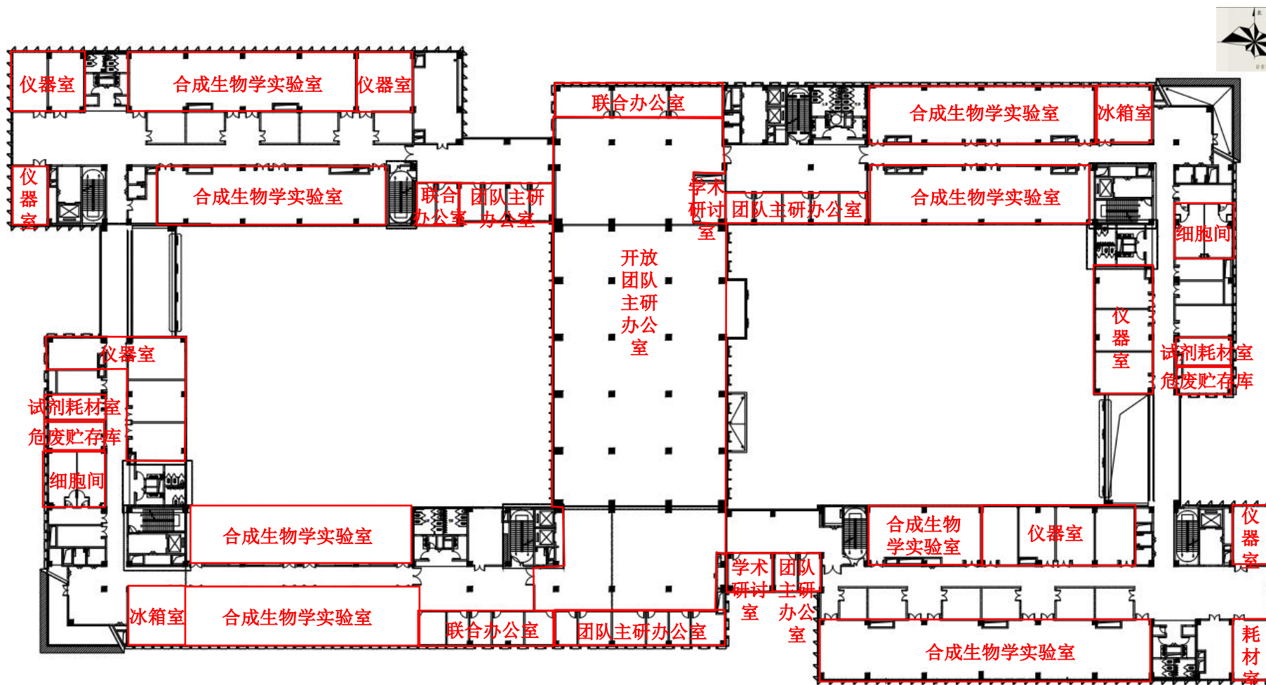
附图 5-4 四层平面布置图 (1:150)
