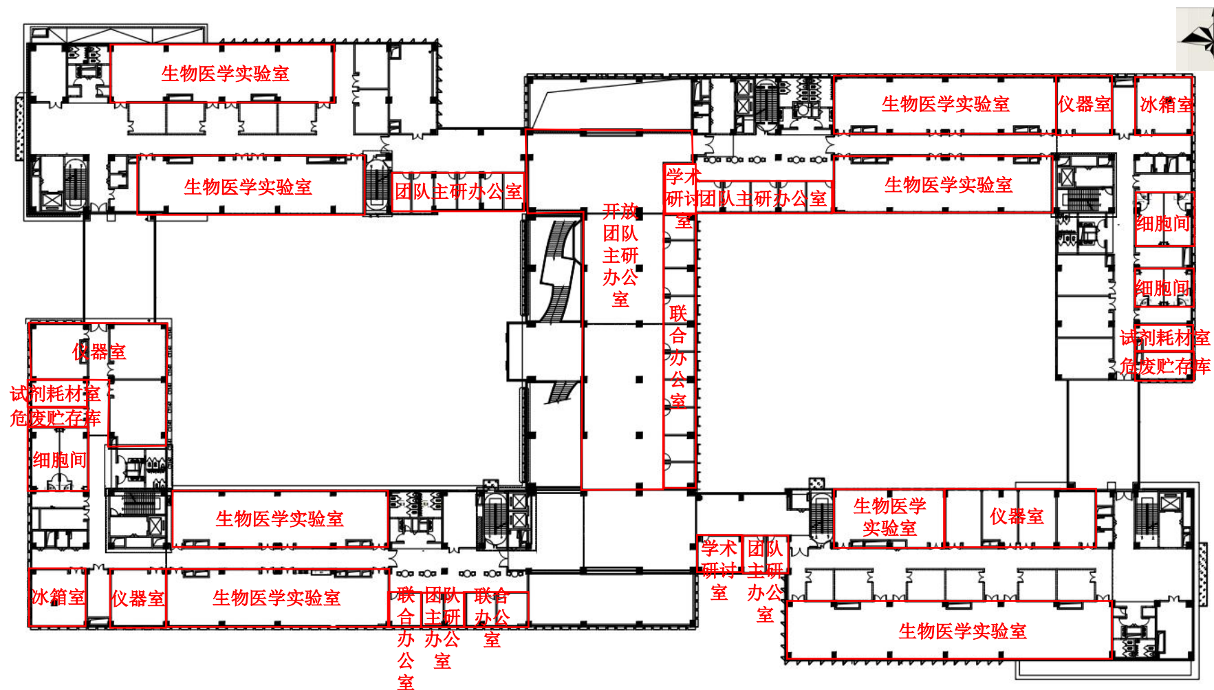
附图 5-2 二层平面布置图 (1:150)
