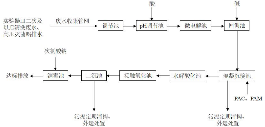
图 4-1 废水处理设备工艺流程图
