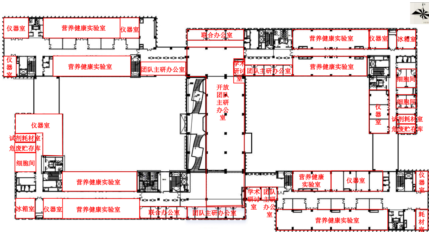
附图 5-3 三层平面布置图 (1:150)
